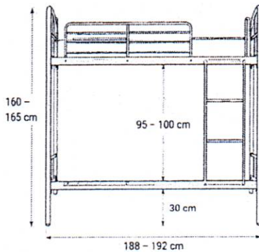
MẶT TRƯỚC
