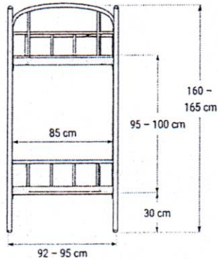
MẶT BÊN
